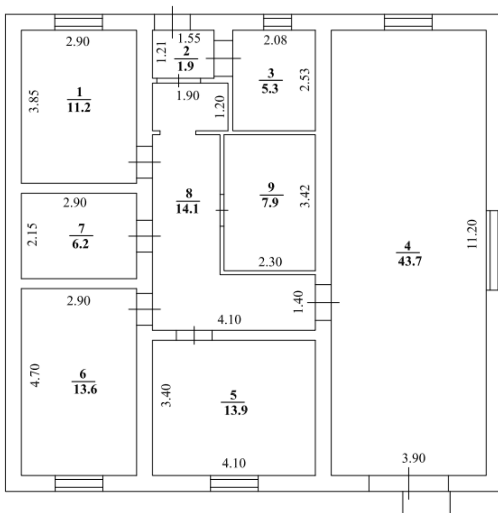
Рис. 12. Поэтажный план здания – объекта кадастровых работ
