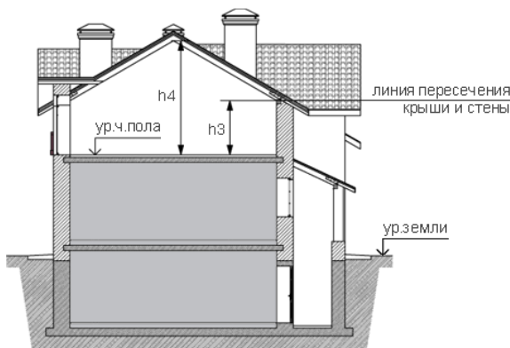
Рис.1. Определение мансардного этажа ( h_3 < 1.5 \text{ м.} )
