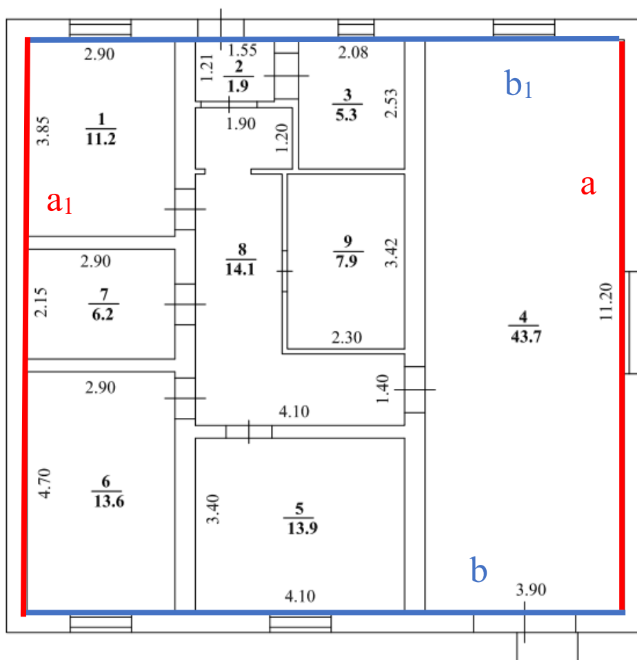
Рис. 16. Линейные измерения для расчета СКП площади здания
