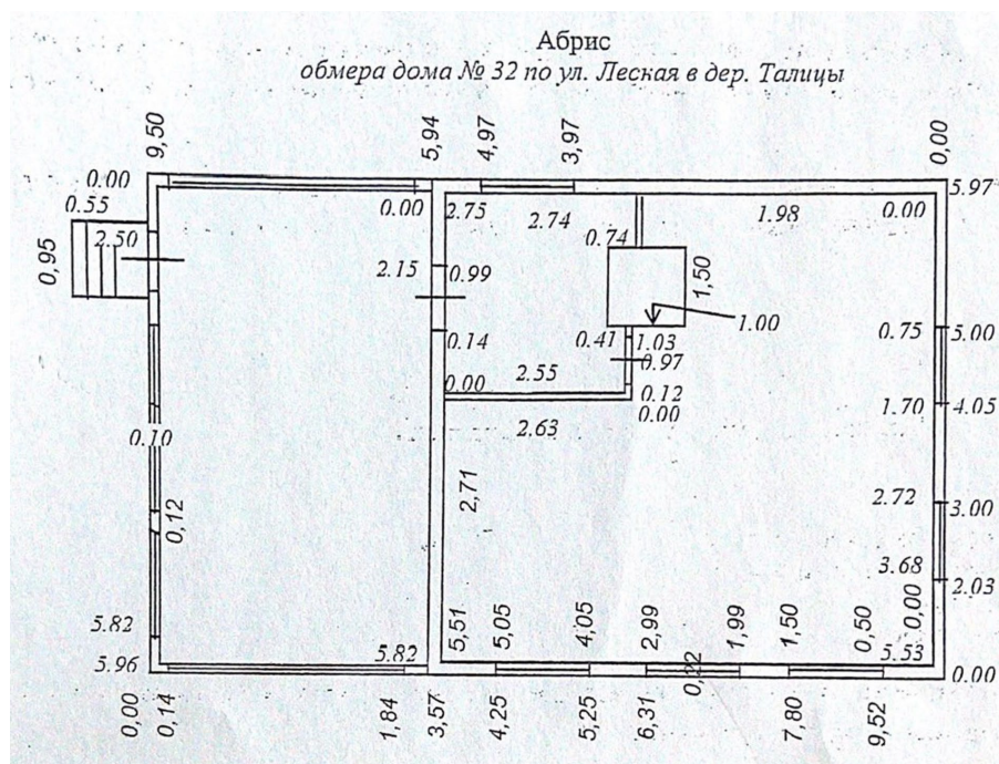
Рис. 22. Пример абриса жилого дома, оформленного посредством автоматизированных средств
