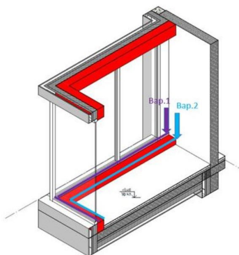
Рис. 8. Особенности подсчета площади помещения при наличии напольных систем отопления.
