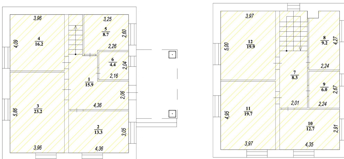
Рис. 7. Подсчет площади здания в пределах этажа
