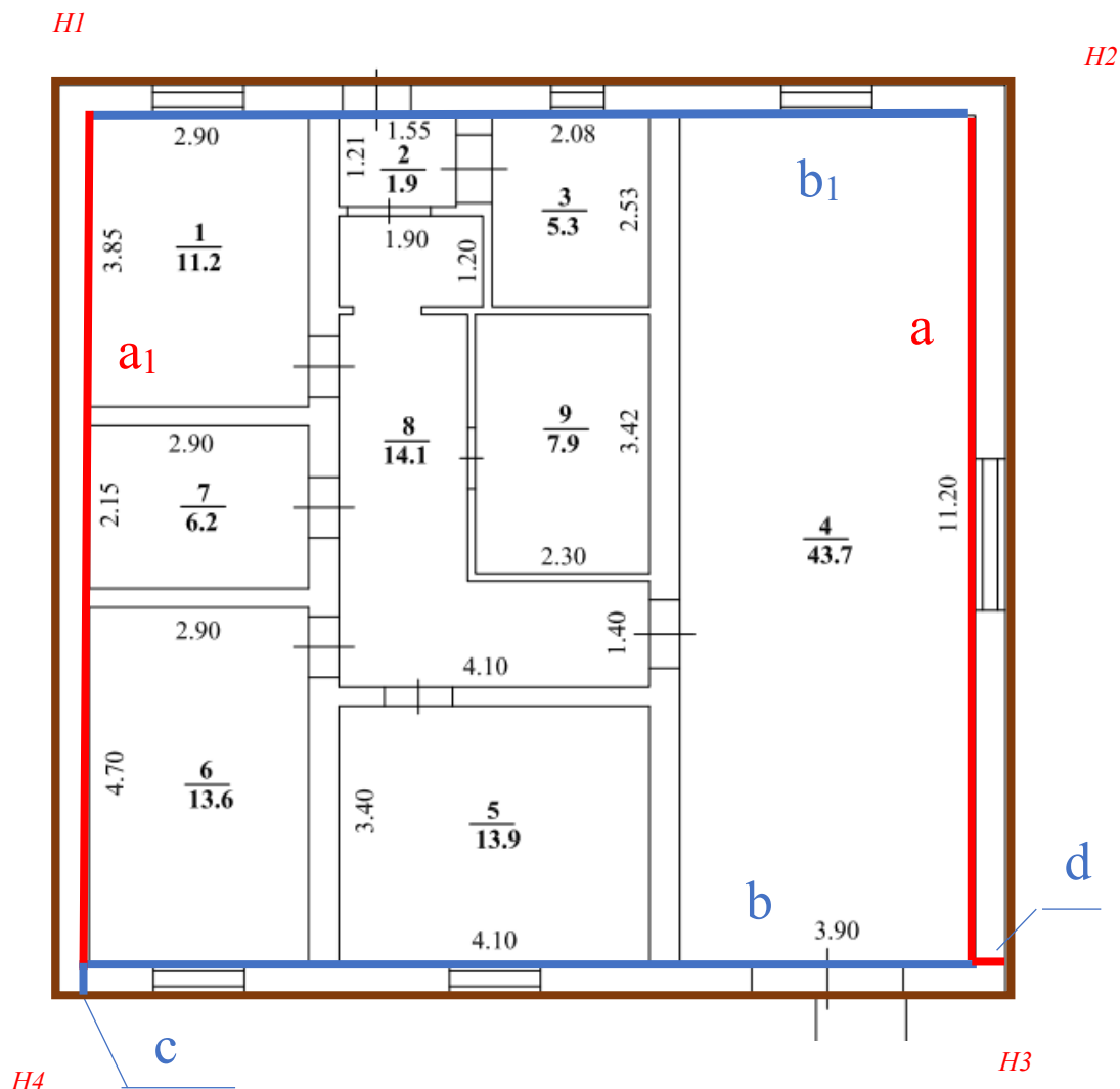
Рис. 17. Линейные измерения для расчета СКП площади здания
