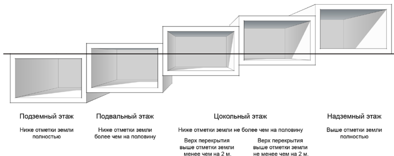
Рис. 5. Сравнение подземного, подвального, цокольного и надземного этажа 1
