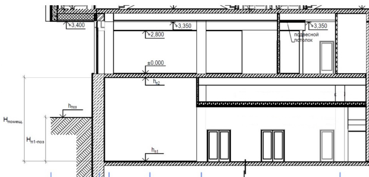
Рис. 4. Определение типа подземного этажа
