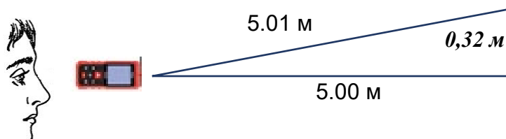
Рис. 14. Определение высоты кривизны лазерного луча
