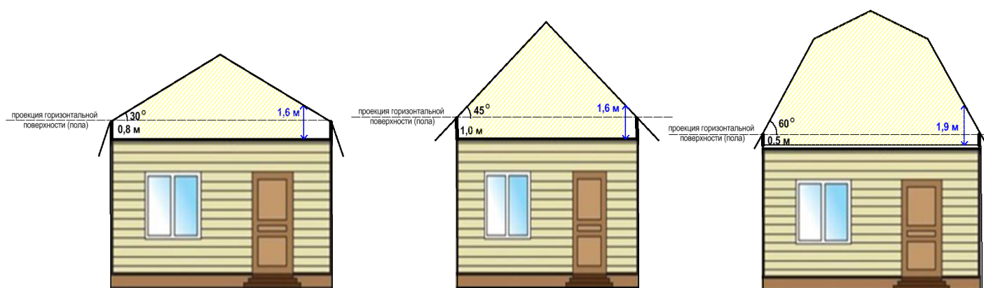
Рис. 11б. Определение площади мансардного этажа жилого здания
